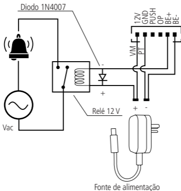
Ligação campainha
