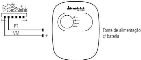
Ligação da fonte de alimentação FA 1220S
