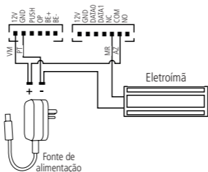
Ligação correta
